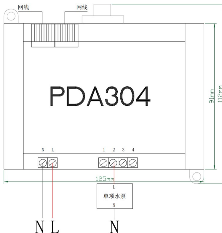
安装及接线示意图
